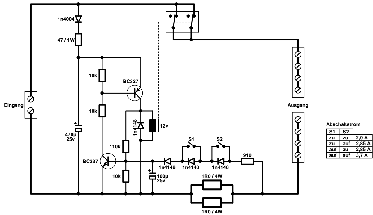
Elektronische Überlast Fahrstromabschaltung (c) Rainer Schroeder
